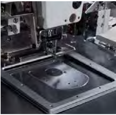
SS 側移壓腳 Side shift clamp
